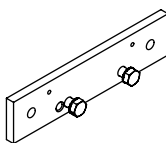
dodatkowa nakładka krokwie 260 × 60 × 12 mm
