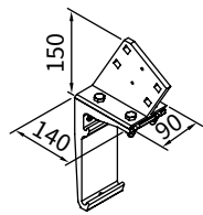
uchwyt krokwiowy 90 mm
