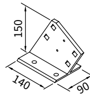
uchwyt krokwiowy nakładka 150 mm
