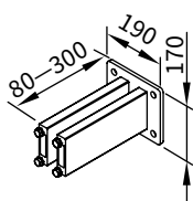
uchwyt dystansowy do 2 uchwyty ściennych 71995.
