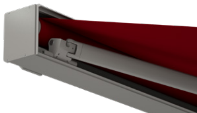
6 podporowe łożysko Rolltex do wałka poszycia, zastosowanie przy dużych szerokościach markiz
