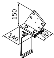
uchwyt krokwiowy 90 mm
