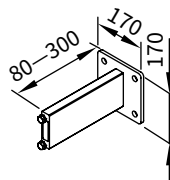
uchwyt dystansowy do uchwyty ściennego 71995.
