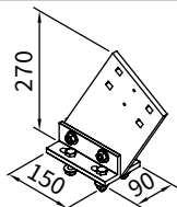
uchwyt krokwiowy 270 mm
